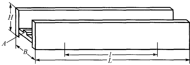
图 2 金属尺
