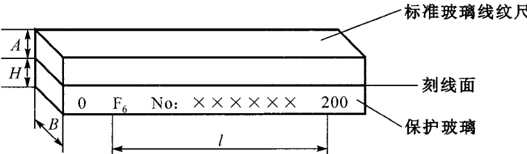
图 1 玻璃尺
