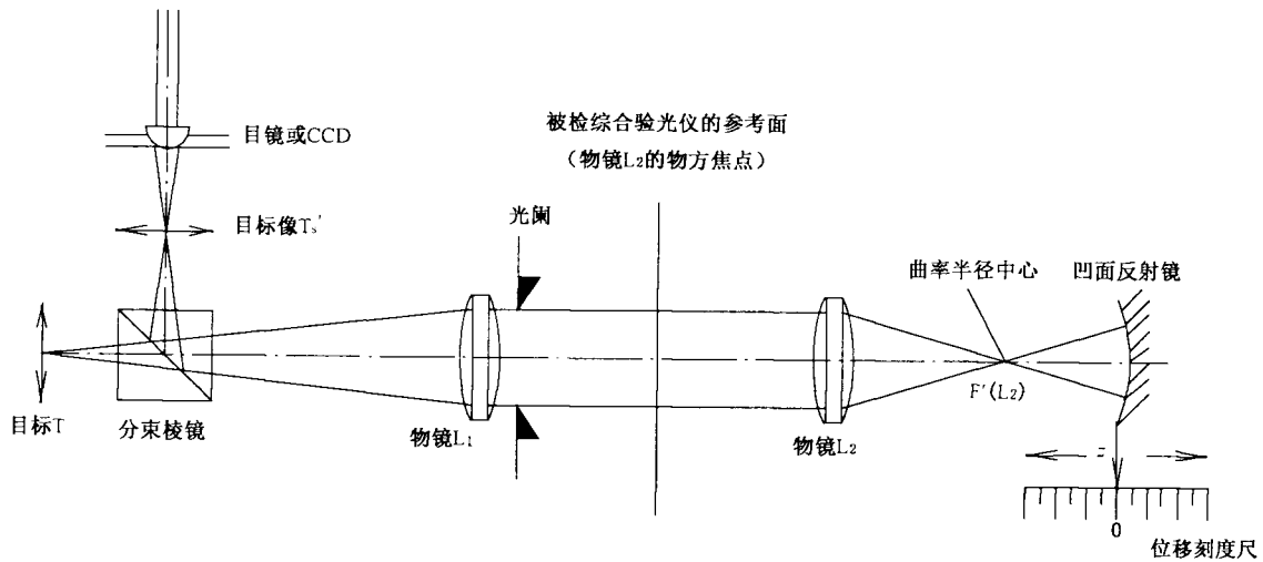
图 C.1 综合验光仪顶焦度测量装置原理示意
